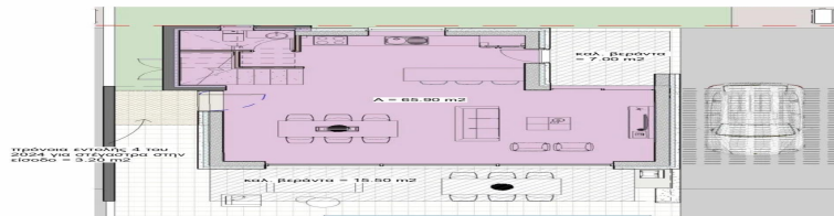
EMBAΔOΓΡΑΜΜΑ ΙΣΟΓΕΙΟΥ_ΚΑΤΟΙΚΙΑ 3 ΚΛΙΜΑΚΑ 1:100
