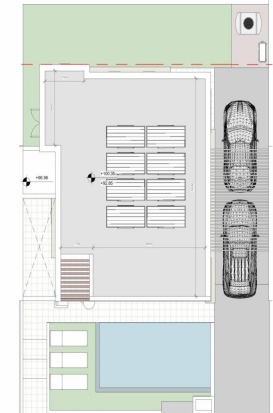
ΚΑΤΩΗ ΟΡΟΦΗΣ_ΚΑΤΟΙΚΙΑ 4 ΚΛΙΜΑΚΑ 1:100
