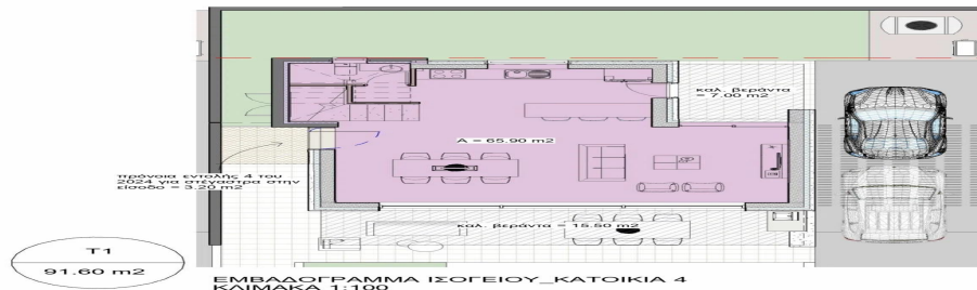
ΕΜΒΑΔΟΓΡΑΜΜΑ ΙΣΟΓΕΙΟΥ_KATOIKIA 4 KΛIΜAKA 1:100
