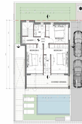
ΚΑΤΩΗ 1ΟΥ ΟΡΟΦΟΥ_ΚΑΤΟΙΚΙΑ 4 ΚΛΙΜΑΚΑ 1:100
