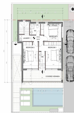
KATONH 1ΟΥ ΟΡΟΦΟΥ_KATOIKIA 4 KΛIΜAKA 1:100
