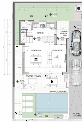
ΚΑΤΩΗ ΙΣΟΓΕΙΟΥ_ΚΑΤΟΙΚΙΑ 4 ΚΛΙΜΑΚΑ 1:100
