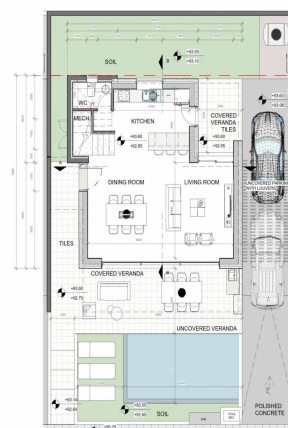
KATONH ISOΓEIOY_KATOIKIA 4 KΛIΜAKA 1:100
