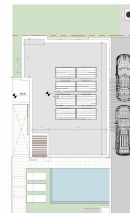
KATONH ΟΡΟΦΗΣ_KATOIKIA 4 KΛIΜAKA 1:100
