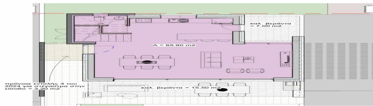
EMBAΔOPAMMA HZOFEIOY_KATOIKIA 5 KAIΜAKA 1:100
