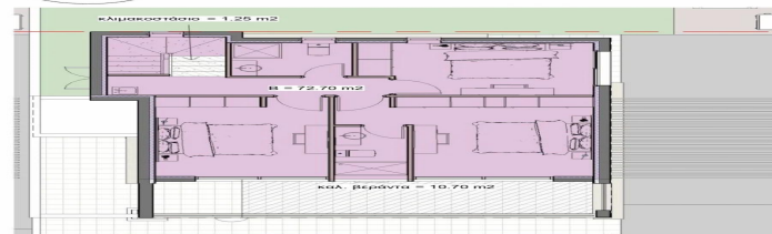
EMBAΔOΓPAMMA 1OY OROFOY_KATOIKIA 5 KAIMAKA 1:100
