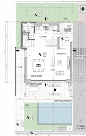
KATOIHI IZOGEIOY_KATOIKIA 5 KAIMAKA 1:100
