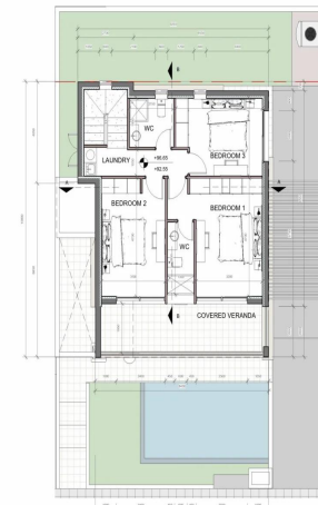
KATOIHI 1OY OROFOY_KATOIKIA 5 KAIMAKA 1:100
