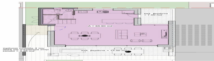
EMBAΔOPAPMA 1OY OROFOYU_KATOIKIA 5 KAIIMAKA 1:100
