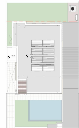
KATOPI OROPHIS_KATOIKIA 5 KAIIMAKA 1:100
