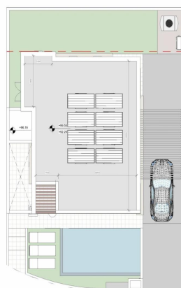
ΚΑΤΩΦΗ ΟΡΟΦΗΣ_ΚΑΤΟΙΚΙΑ 6 ΚΛΙΜΑΚΑ 1:100
