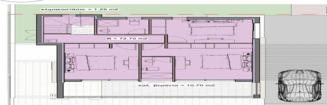
ΕΜΒΛΑΔΟΓΡΑΜΜΑ 1ΟΥ ΟΡΟΦΟΥ_ΚΑΤΟΙΚΙΑ 6 ΚΛΙΜΑΚΑ 1:100
