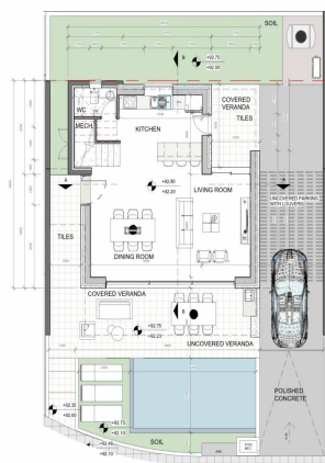
ΚΑΤΩΦΗ ΙΣΟΓΕΙΟΥ_ΚΑΤΟΙΚΙΑ 6 ΚΛΙΜΑΚΑ 1:100
