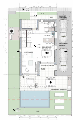
KATOIHI IZOΓEIOY_KATOIKIA 11 ΚΑΙΜΑΚΑ 1:100
