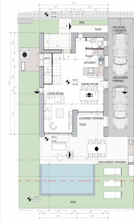
KATOIHI IZOΓEIOY_KATOIKIA 11 KΛIΜAKA 1:100
