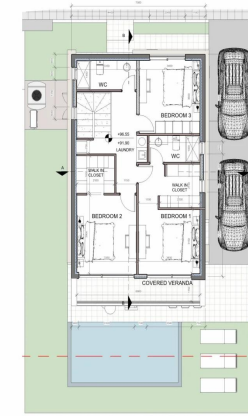
KATOIHI 1ΟΥ ΟΡΟΦΟΥ_KATOIKIA 11 KΛIΜAKA 1:100
