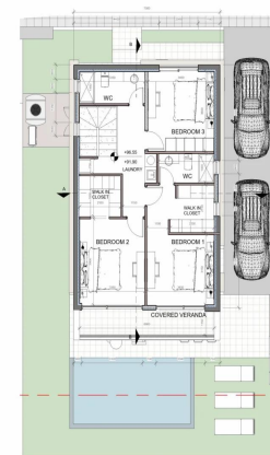
KATOIHI 1ΟΥ ΟΡΟΦΟΥ_KATOIKIA 11 ΚΑΙΜΑΚΑ 1:100
