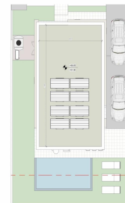
KATOIHI ΟΡΟΦΗΣ_KATOIKIA 11 ΚΑΙΜΑΚΑ 1:100
