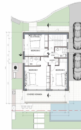
KATOWH 1OY OPOΦOY_KATOIKIA 12 KAIMAKA 1:100
