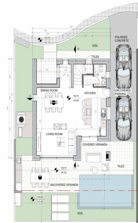
KATOWH IZOFIOY_KATOIKIA 12 KAIMAKA 1:100
