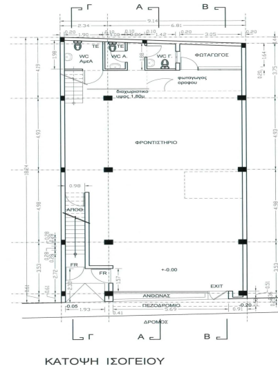
ΚΑΤΟΨΗ ΙΣΟΓΕΙΟΥ
