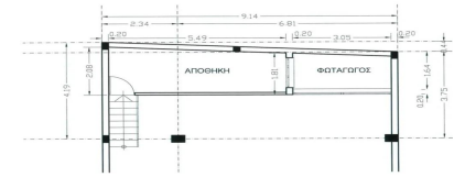
ΚΑΤΟΨΗ ΠΑΤΑΡΙΟΥ
