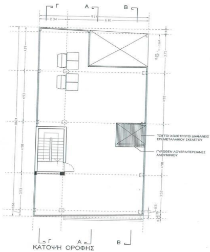
ΚΑΤΟΨΗ ΟΡΟΦΗΣ
