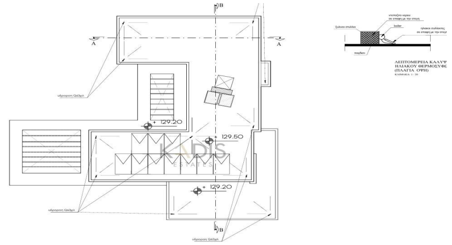
ΚΑΤΟΙΚΙΑ 1 ΚΑΤΩΦΗ ΟΡΟΦΗΣ ΚΛΙΜΑΚΑ 1:100
