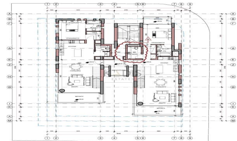
ΚΑΤΩΦΗ ΕΠΙΠΕΔΟ 9 (ΔΙΟΡΘΩΦ ΔΙΑΜΕΡΙΣΜΑ 3 ΥΠΝΟΔΟΜΩΜΑΤΩΝ ΚΑΤΩΤΕΡΟ ΕΠΙΠΕΔΟ)
