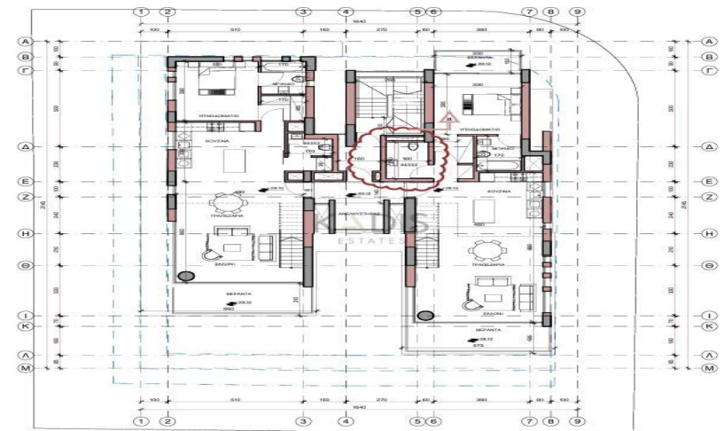
ΚΑΤΩΦΗ ΕΠΙΠΕΔΟ 0 (ΔΙΟΡΘΩΣΗ ΔΙΑΜΕΤΡΙΣΜΑ 3 ΥΠΝΟΔΟΜΑΤΙΩΝ ΚΑΤΩΤΕΡΟ ΕΠΙΠΕΔΟ)
