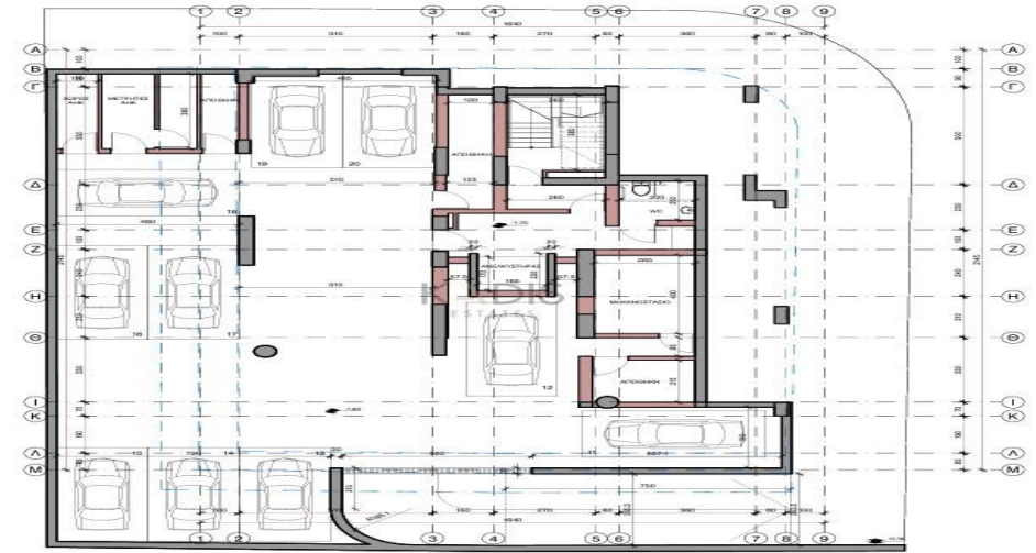
ΚΑΤΩΦΗ ΥΠΟΓΕΙΟΥ
