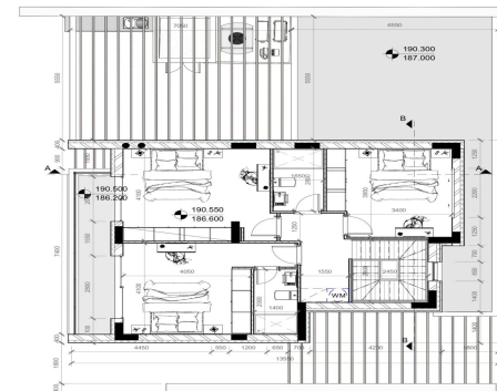
Κατοικία 5 Κότιση αρχικού Καλυμνία 1.100 Εμβαδόν = 88,5 τ.μ
