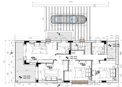
Κατοικία 6 Κλίση ορόφου Κλίση 1:100 Εμβαδόν = 98.01 μ²
