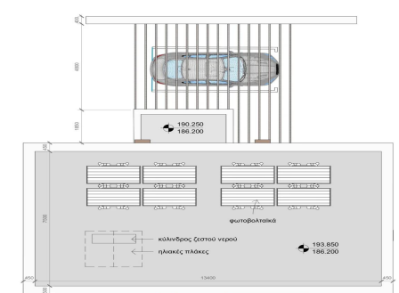
Κατοικία 6 Κλίση ορόφου Κλίση 1:100
