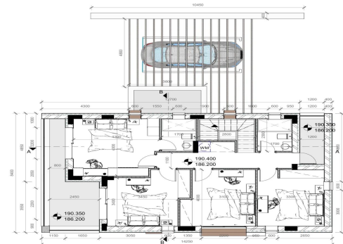
Κατοικία 6 Καθαρή ορόσηνη Καθαρότητα 1100 Εμβαδόν = 96.01 μ²
