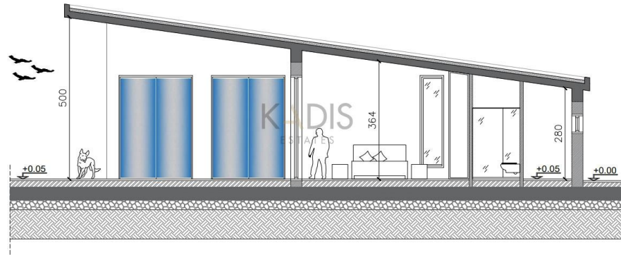
ΤΟΜΗ ΑΑ' - ΚΥΡΙΑ ΚΑΤΟΙΚΙΑ ΚΑΙΜΑΚΑ 1/50
