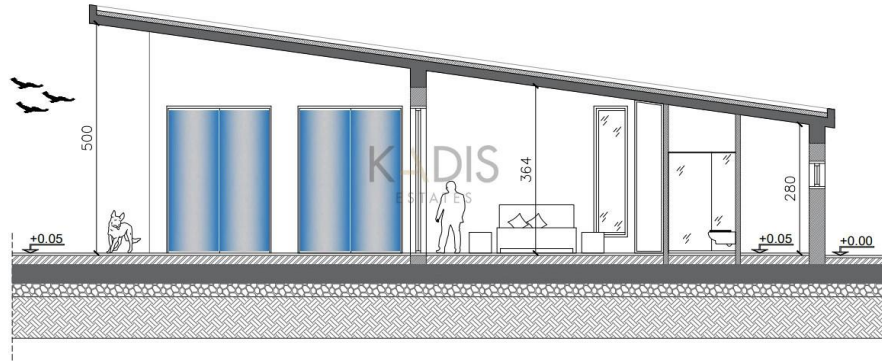
TOMH AA' - KYPIA KATOIKIA KΛΙΜΑΚΑ 1/50
