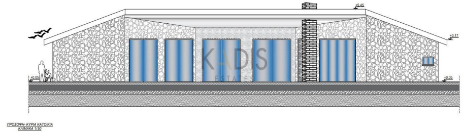
ΠΡΟΣΩΠΗ ΚΥΡΙΑ ΚΑΤΟΙΚΙΑ ΚΛΙΜΑΚΑ 1/50
