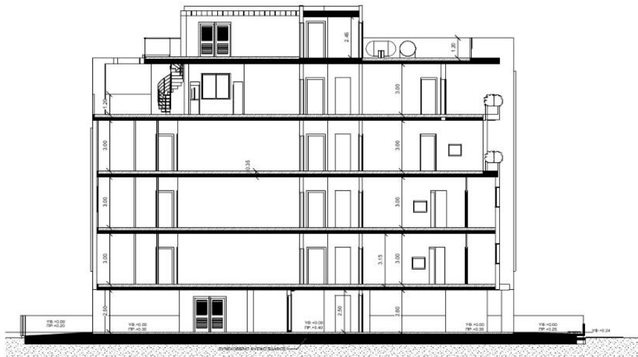
1 ΤΟΜΗ 1/A111 1:100
