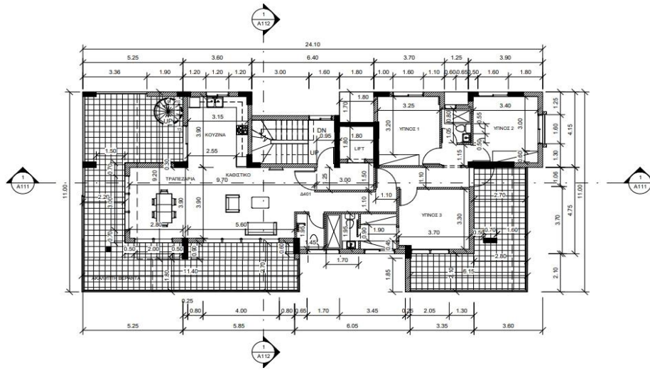
1 ΚΑΤΩΦΗ 4ου ΟΡΟΦΟΥ 1:100
