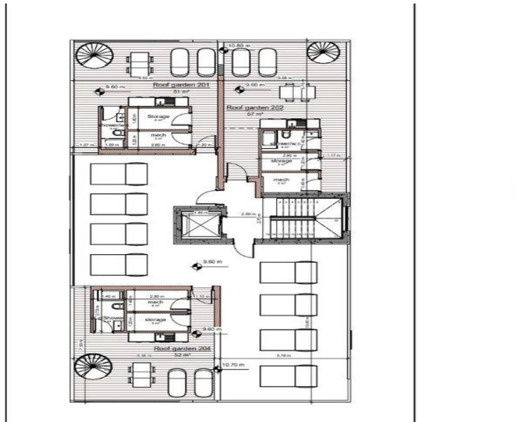
1 Roof garden 1 : 100
