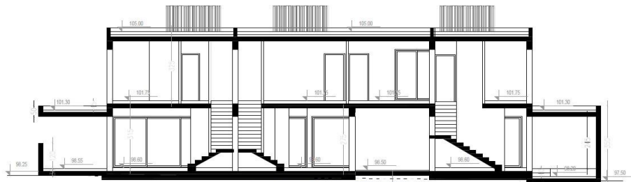
KATOIKIA 01+02+03 TOMH B-B
