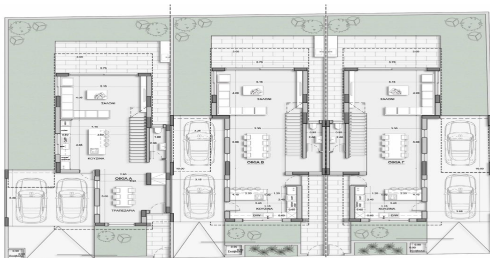
ΚΑΤΟΨΗ ΙΣΟΓΕΙΟΥ
