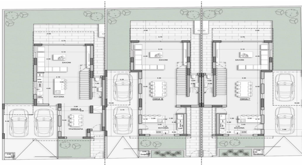
ΚΑΤΟΨΗ ΙΣΟΓΕΙΟΥ
