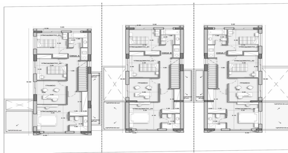
ΚΑΤΟΨΗ ΟΡΟΦΟΥ
