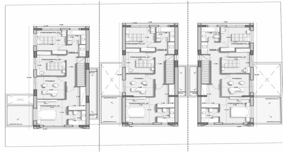
ΚΑΤΟΨΗ ΟΡΟΦΟΥ
