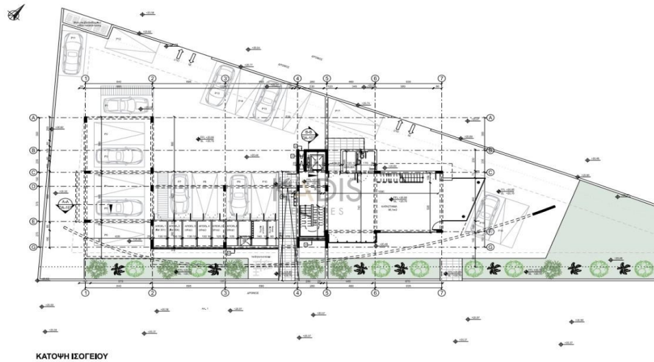
ΚΑΤΟΧΗ ΙΣΟΓΕΙΟΥ
