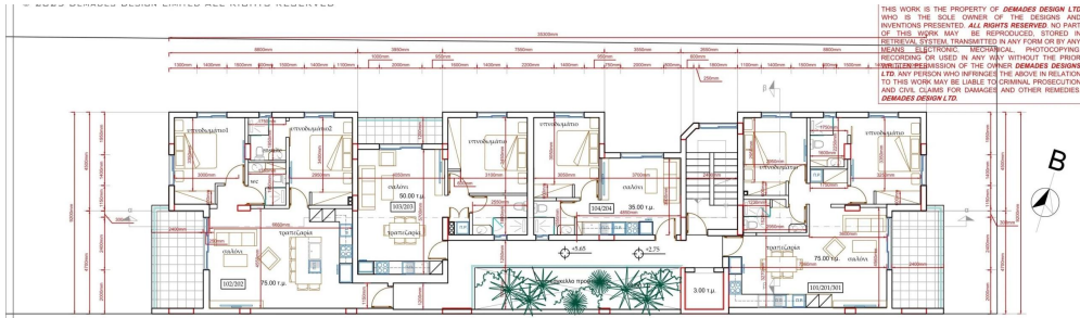
Κάτοψη 1ου & 2ου ορόφου
