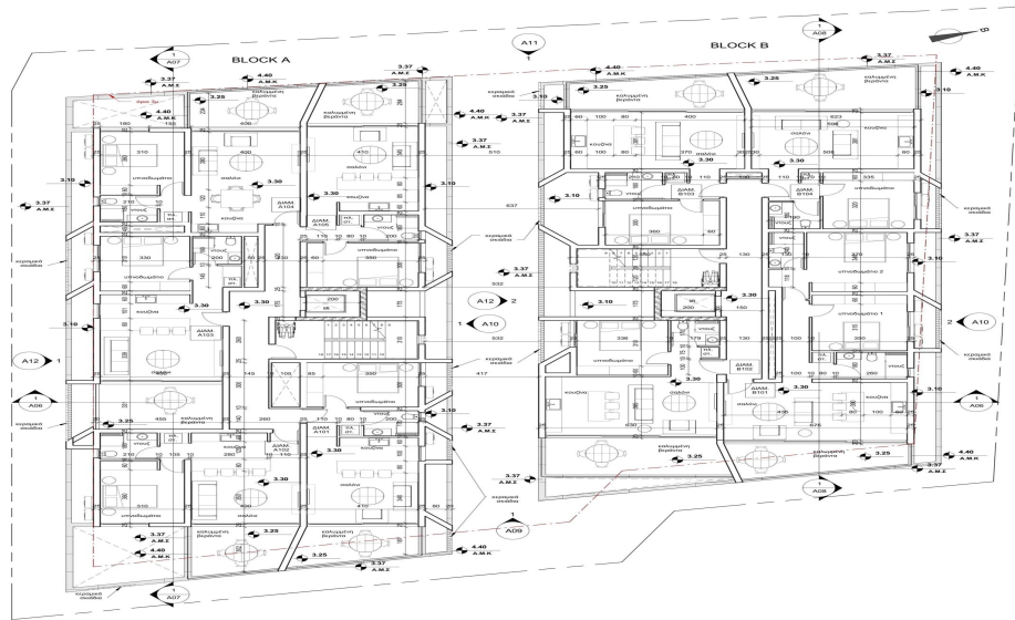
1 02 - Κάτοψη 1ου Ορόφου 1:100
