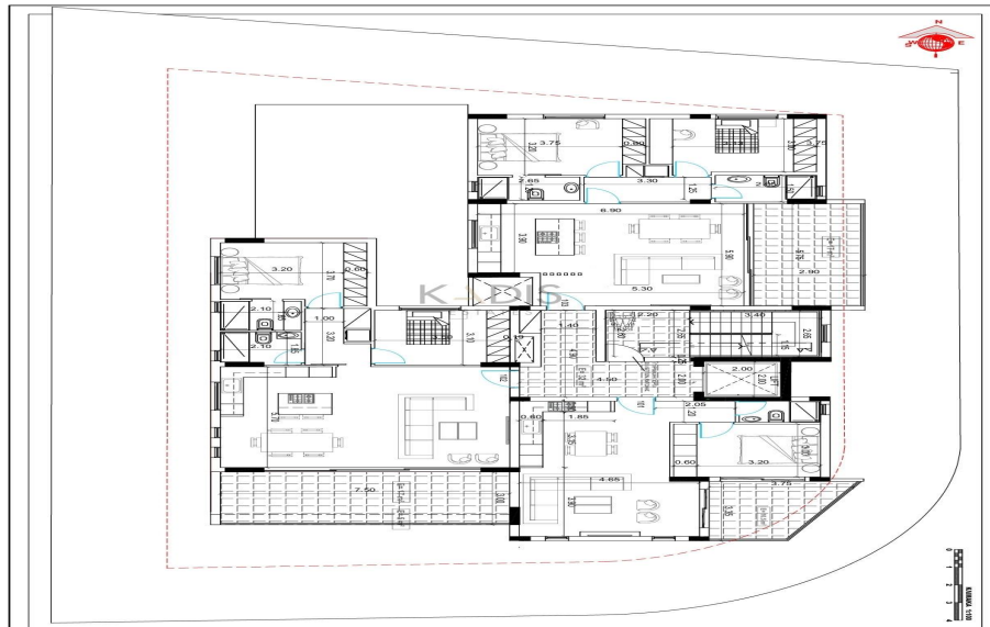
ΚΑΤΟΨΗ 1ου ΟΡΟΦΟΥ
