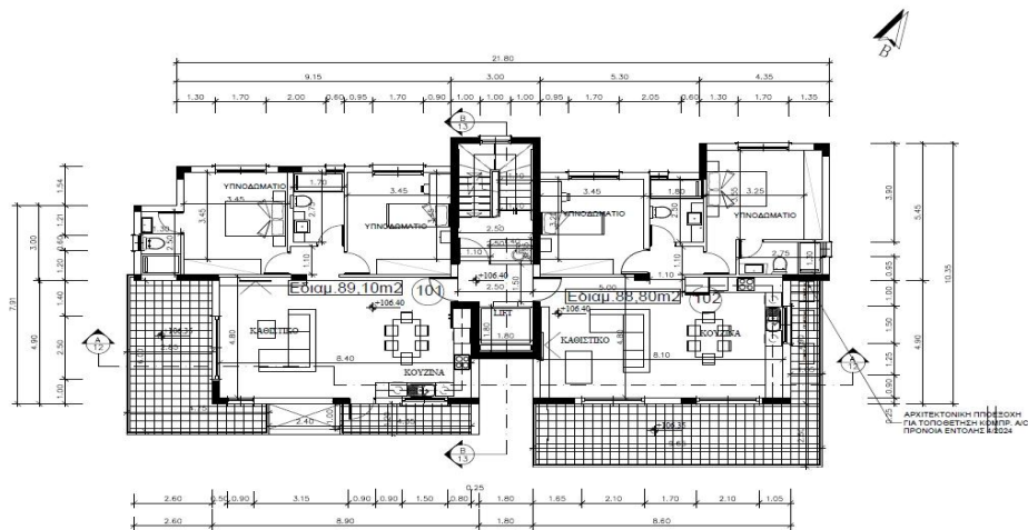
ΚΑΤΩΦΗ 1ου ΟΡΟΦΟΥ ΚΛΙΜΑΚΑ 1:100
