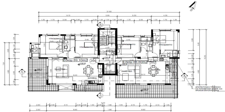
ΚΑΤΩΦΗ 2ου ΟΡΟΦΟΥ ΚΛΙΜΑΚΑ 1:100
