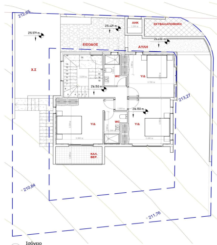
1 Ισόγειο 1 : 100
