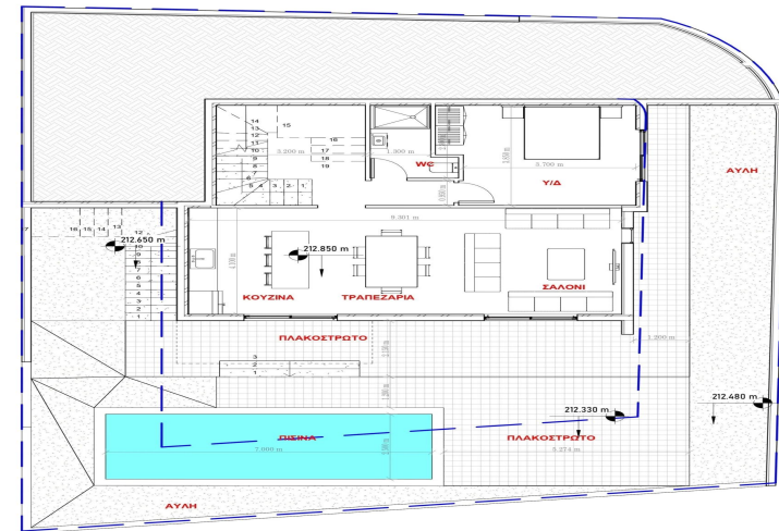
1 Υπόγειο 1 : 100
