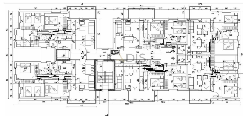
Κάτοψη ορόφου 4 1:100
