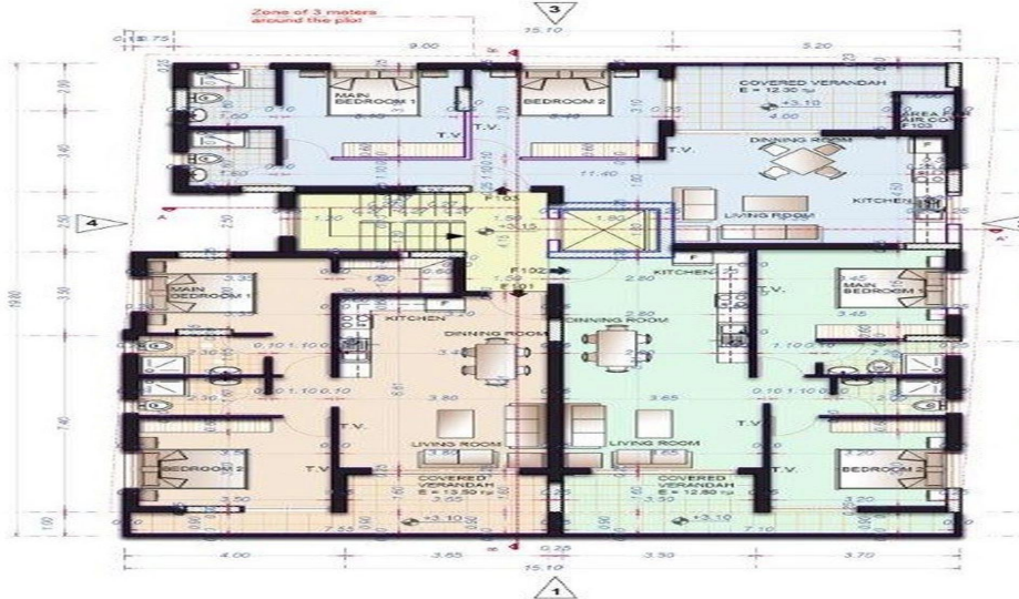
1st FLOOR PLAN ΚΑΤΟΨΗ 1ου ΟΡΟΦΟΥ ΚΛΙΜΑΚΑ 1:100
