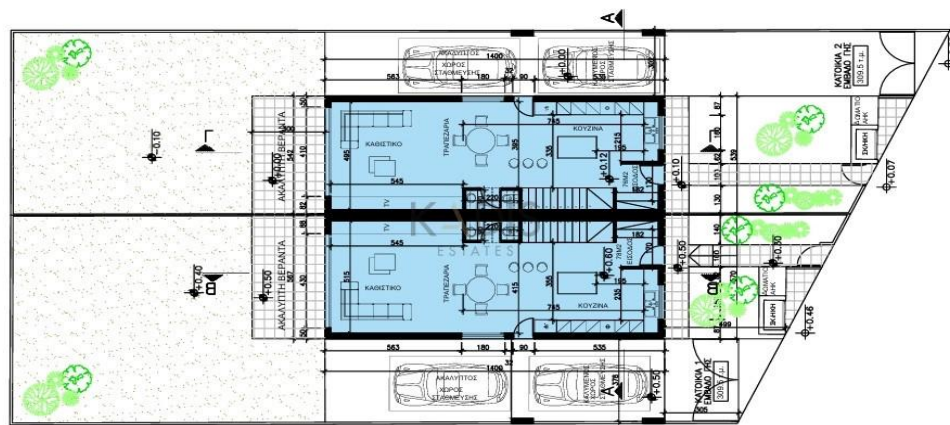
T1 154m 2 ΚΑΤΟΠΗ ΙΣΟΓΕΙΟΥ
