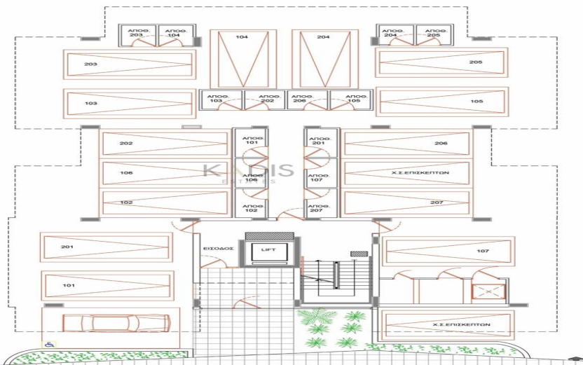
Κάτοψη Ισογείου
