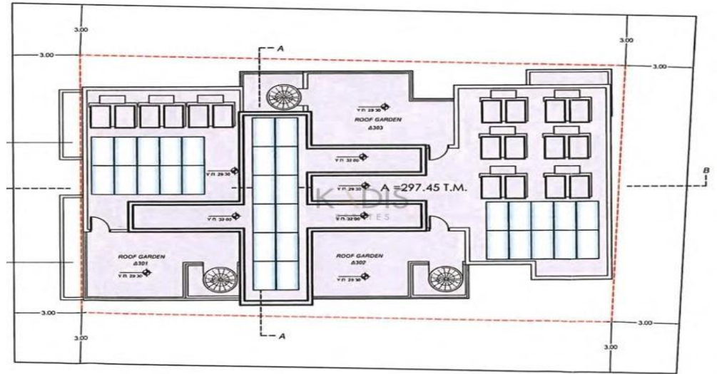
ΚΑΤΟΨΗ ΔΩΜΑΤΟΣ κλίμακα 1/200
