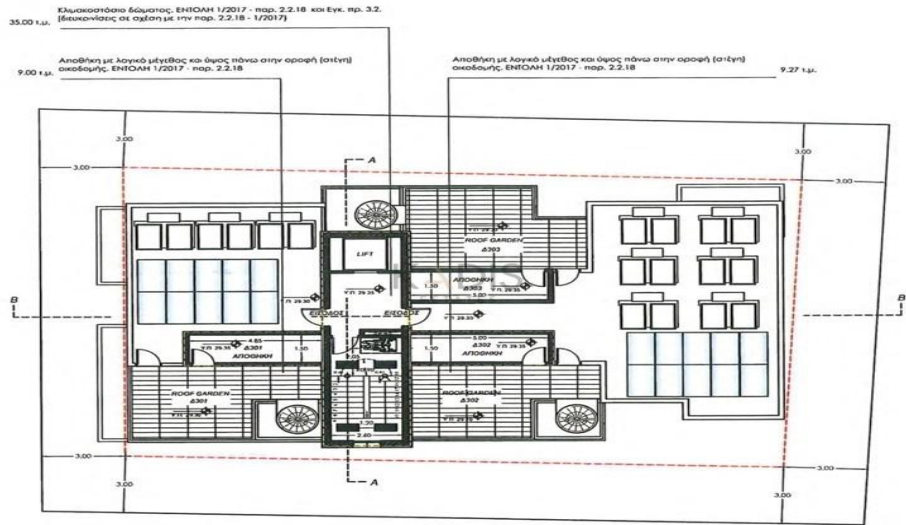
ΚΑΤΟΨΗ ΟΡΟΦΗΣ - ROOF GARDEN κλίμακα 1/200
