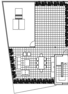
ΚΑΤΩΦΗ ΟΡΟΦΗΣ (κλ. 1-100)
