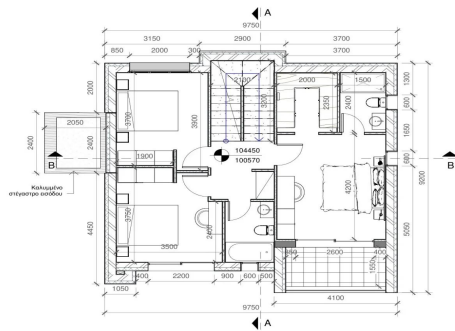
Κατοικία 7 Κάτοψη ορόφου Κλίμακα 1:100 Εμβαδόν= 74.70 τ.μ.
