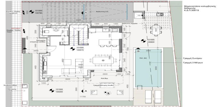
Κατοικία 7 Κάτοψη ισόγειου Κλίμακα 1:100 Εμβαδόν= 72.30 τ.μ.
