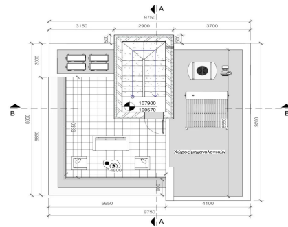
Κατοικία 7 Κάτοψη οροφής Κλίμακα 1:100
