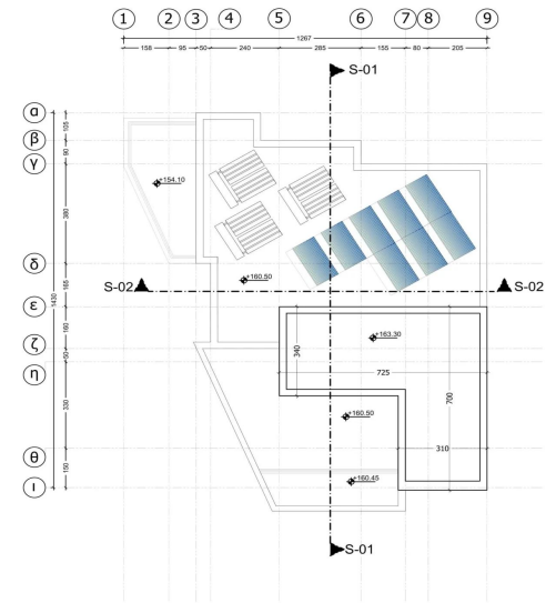
κατοψη οροφης κλίμακα 1 / 100
