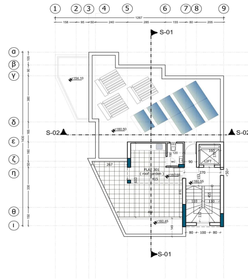
κατοψη οροφης ( roof garden ) κλίμακα 1 / 100
