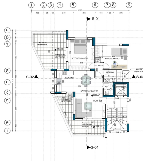
κατοψη 2ου οροφου κλίμακα 1 / 100
