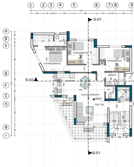
κατοψη 1ου οροφου κλίμακα 1 / 100
