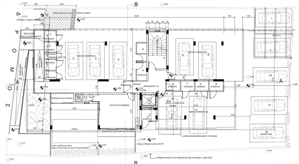
ΚΑΤΟΧΗ ΙΣΟΓΕΙΟΥ
