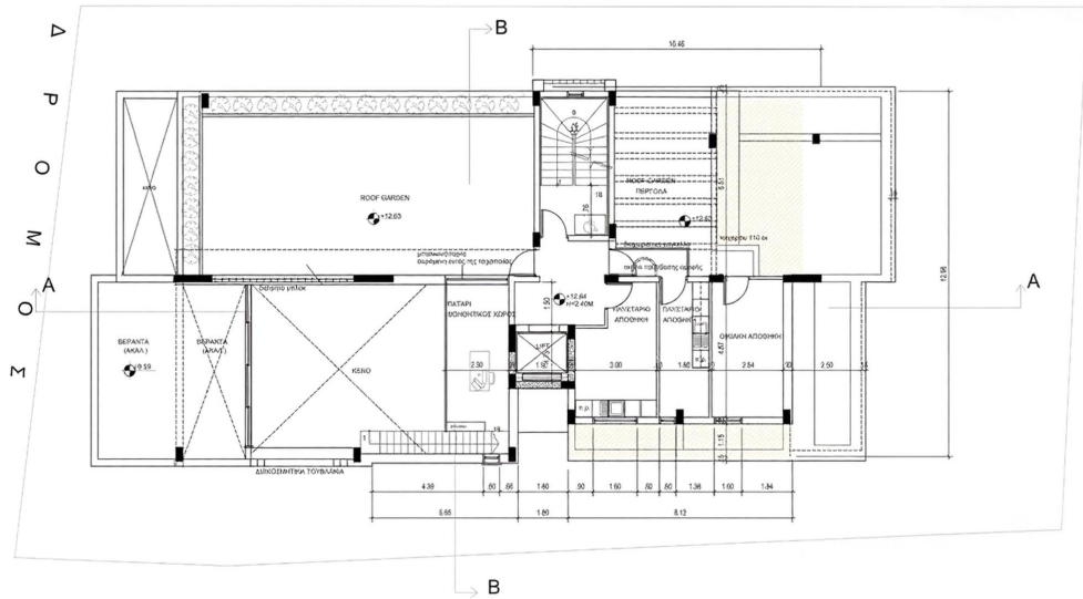
ΚΑΤΟΧΗ ΟΡΟΦΗΣ
