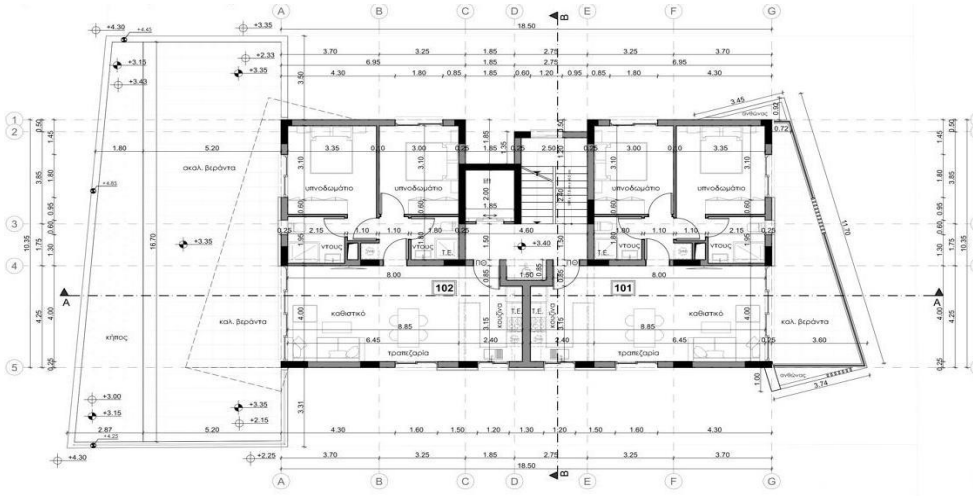
ΚΑΤΩΦΗ 1-ου ΟΡΟΦΟΥ 1:100
