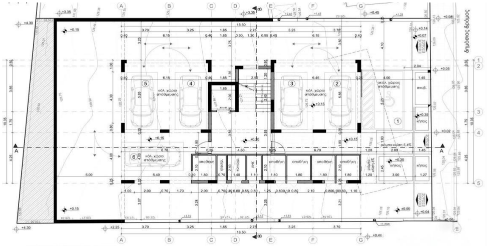
ΚΑΤΩΦΗ ΙΣΟΓΕΙΟΥ / ΧΩΡΟΤΑΞΙΚΟ 1:100
