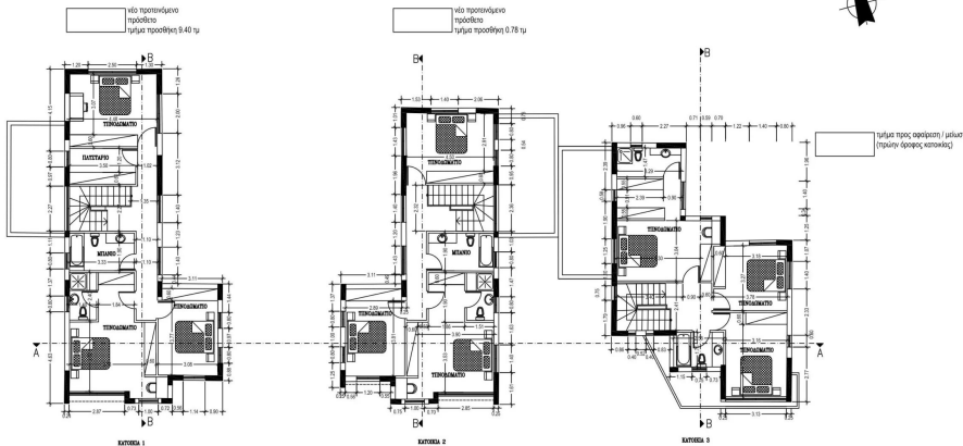
ΚΑΤΟΠΗ ΟΡΟΦΟΥ ΚΑΤΟΙΚΙΑ 1 & 2 & 3
