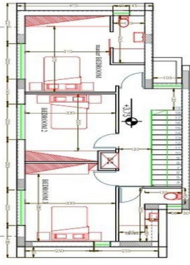
Χωροταξικό-Κατοχή Ισογείου
