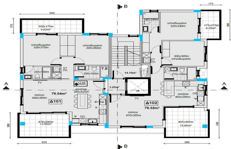
ΚΑΤΟΨΗ 1ου ΟΡΟΦΟΥ ΚΛΙΜΑΚΑ - 1:100
