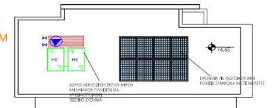
Κατοψη οροφης
