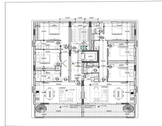
ΚΑΤΩΦΛΙΣΤΙΚΟ ΓΕΩΜΕΤΡΟ
